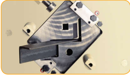
Standaard messen voor L, \emptyset en \nabla .
